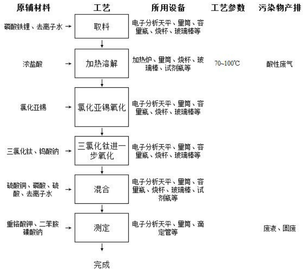
图 2-1 项目锂电池正极材料废液中铁的测定工艺流程图
