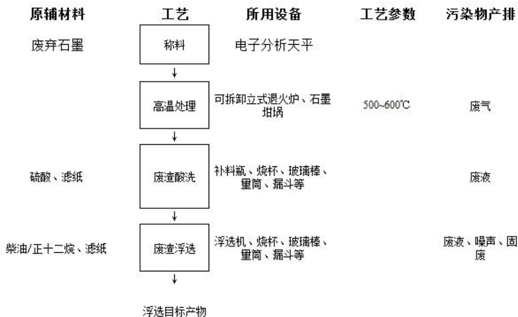
图 2-3 项目研发工艺流程图
