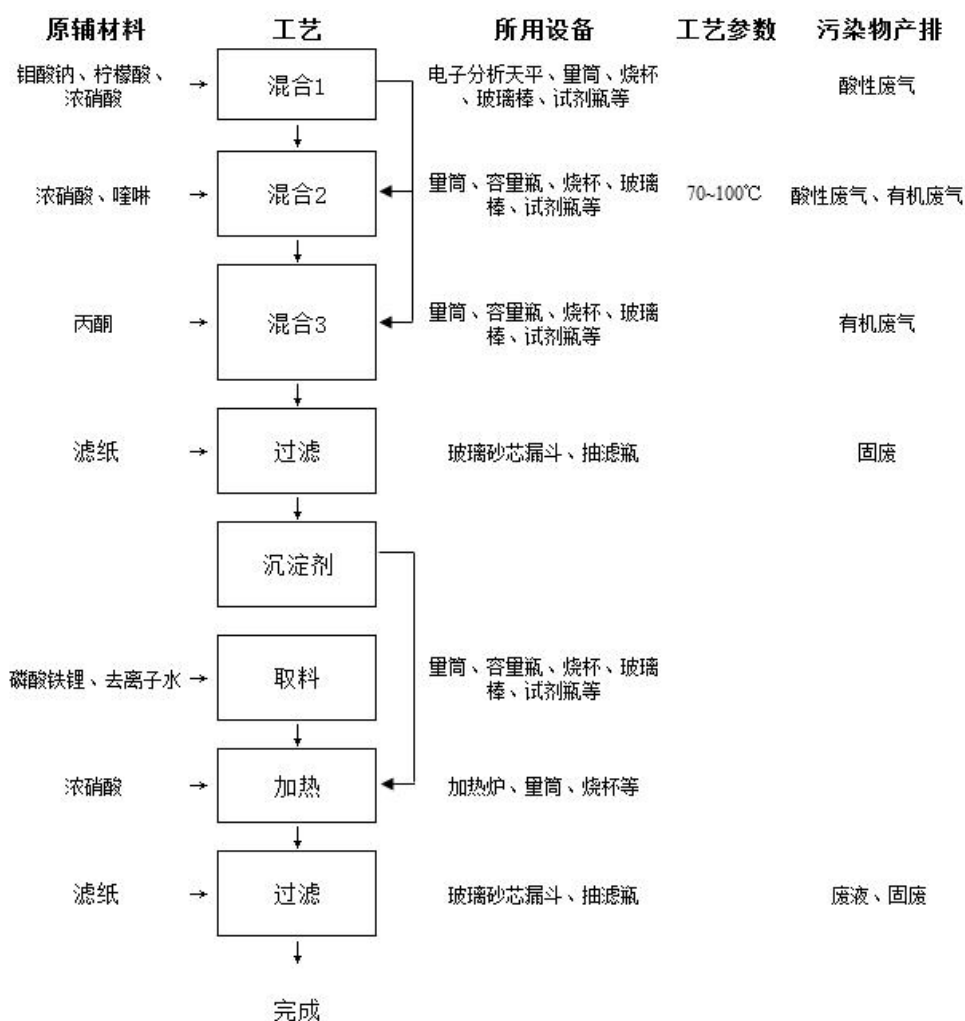
图 2-2 项目锂电池正极材料废液中磷的测定工艺流程图
