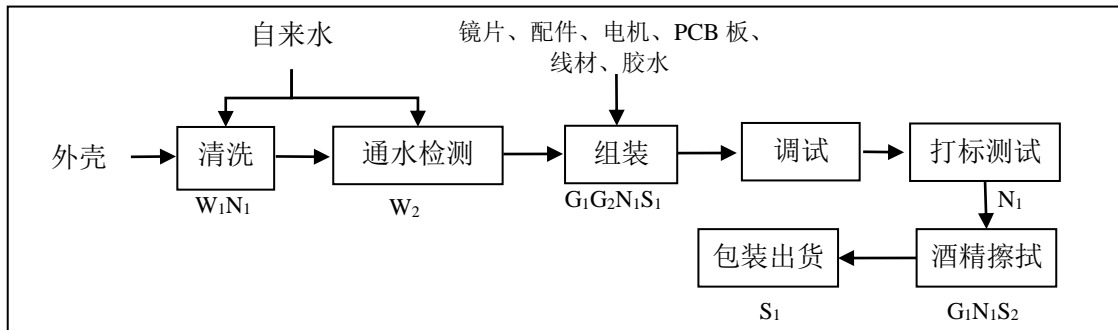
图 2-1 生产工艺流程图 1
