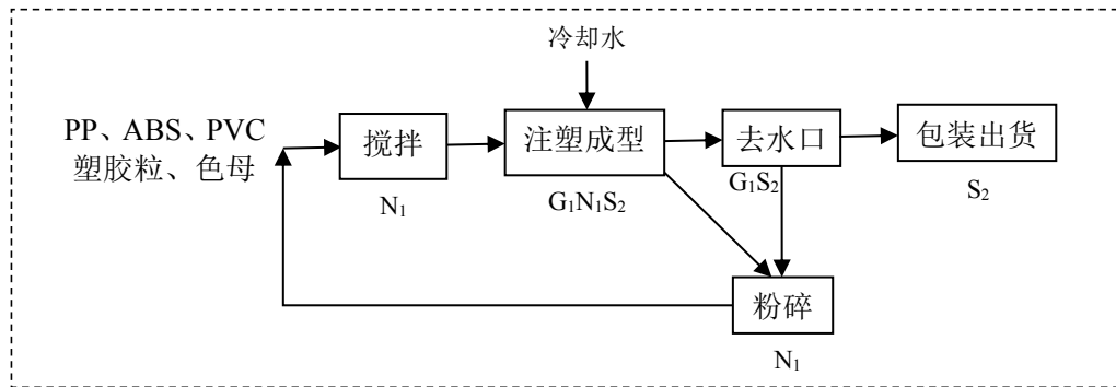
图 2-1 生产工艺流程图
