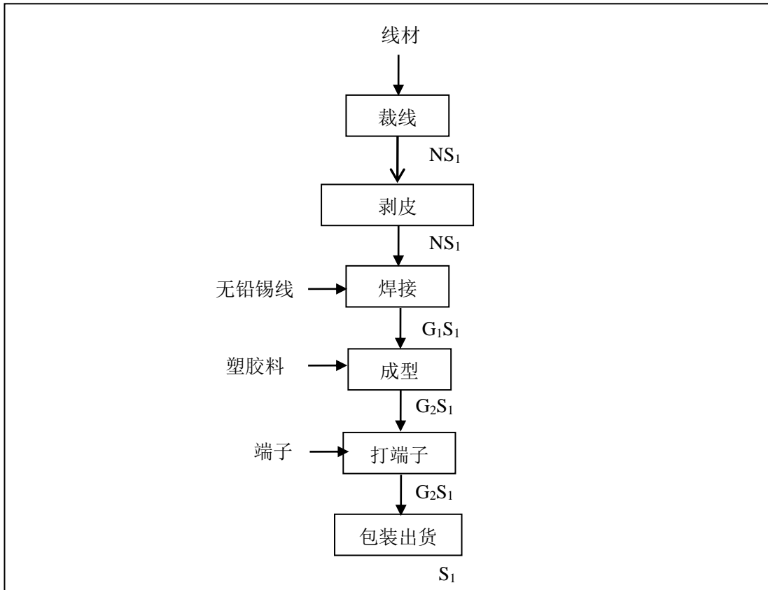
图 6-1 项目生产工艺流程图
