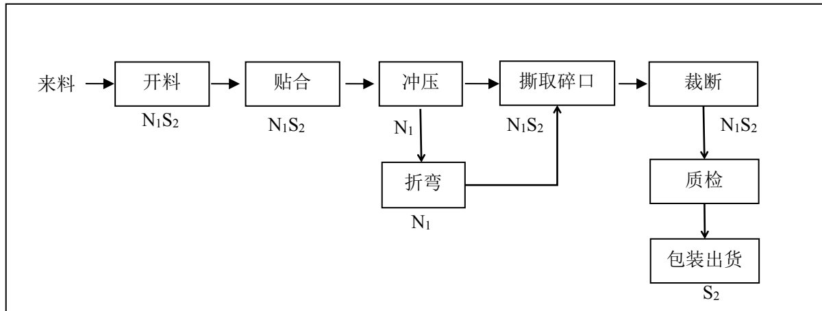
图3 生产工艺流程图
